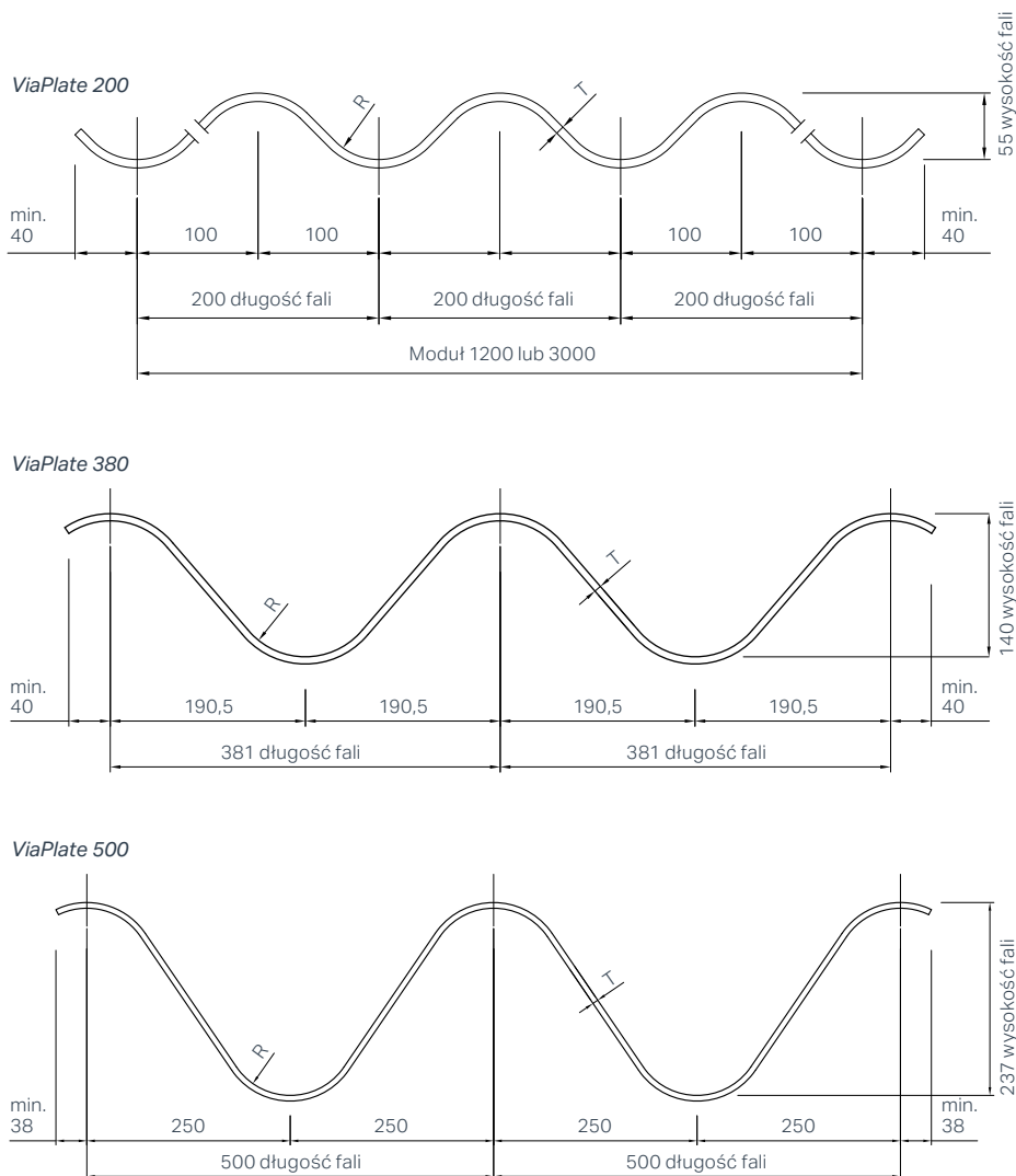
Rys. 1. Przekroje poprzeczne blach ViaPlate.
