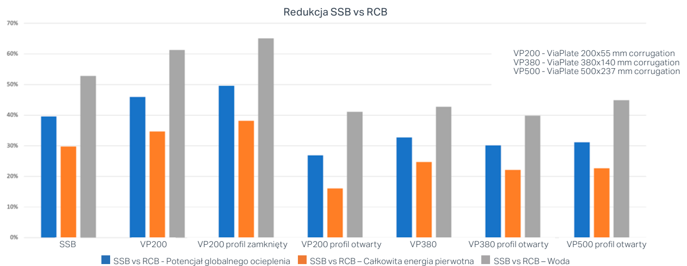
Wykres 1. Analiza porównawcza LCA (cyklu życia produktu) między mostami gruntowo-powłokowymi (SSB - Soil Steel Bridges) wykonanymi z blachy falistej a mostami żelbetowymi (RCB - Reinforced Concrete Bridges).
