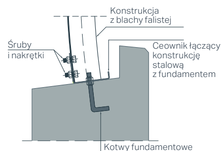
Rys. 7. Połączenie konstrukcji stalowej z fundamentem.
