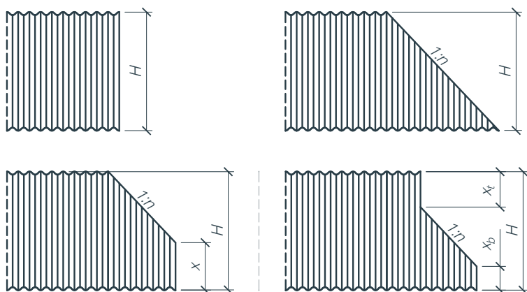
Rys. 4. Zakończenie konstrukcji w przekroju podłużnym.
