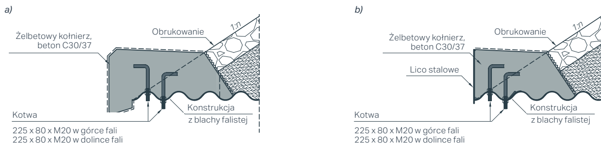
Rys. 6. Przykład wieńca żelbetowego: a) z kapinosem, b) z licem stalowym
