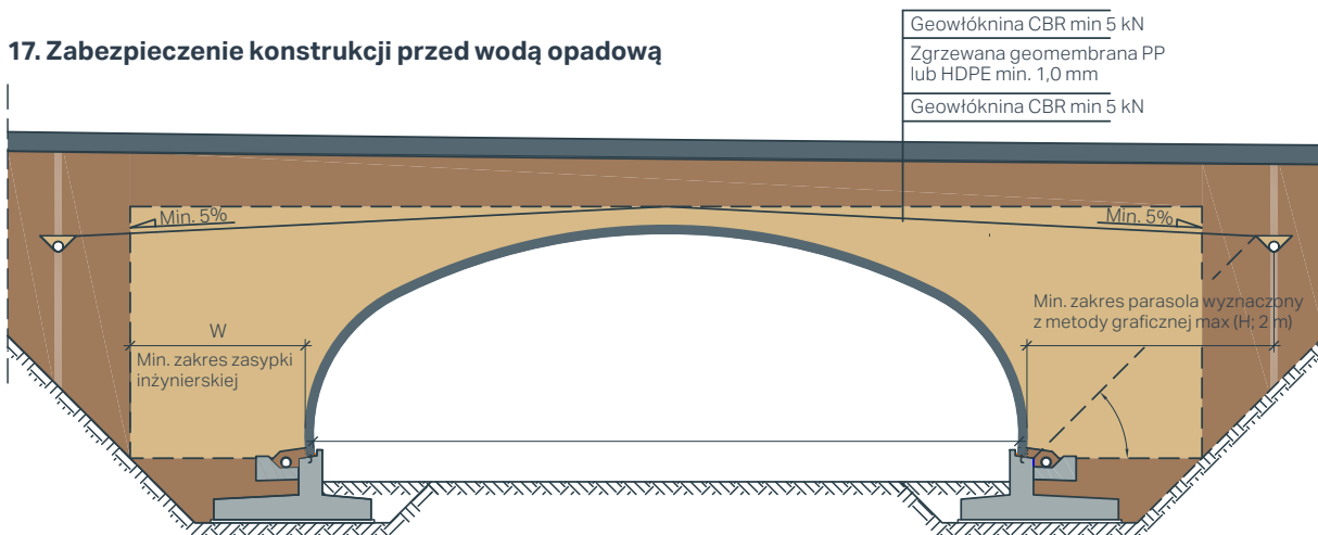
Rys. 8. Schemat zabezpieczenia konstrukcji przed wodą opadową – "parasol" ochronny.
